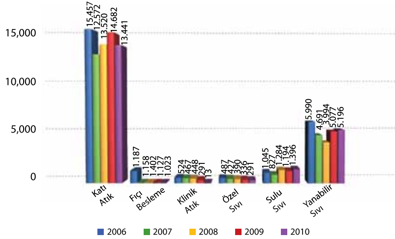
2006 - 2010 Yılları Arasındaki Yakma Tesisinde Yakılan Atık Miktarları
