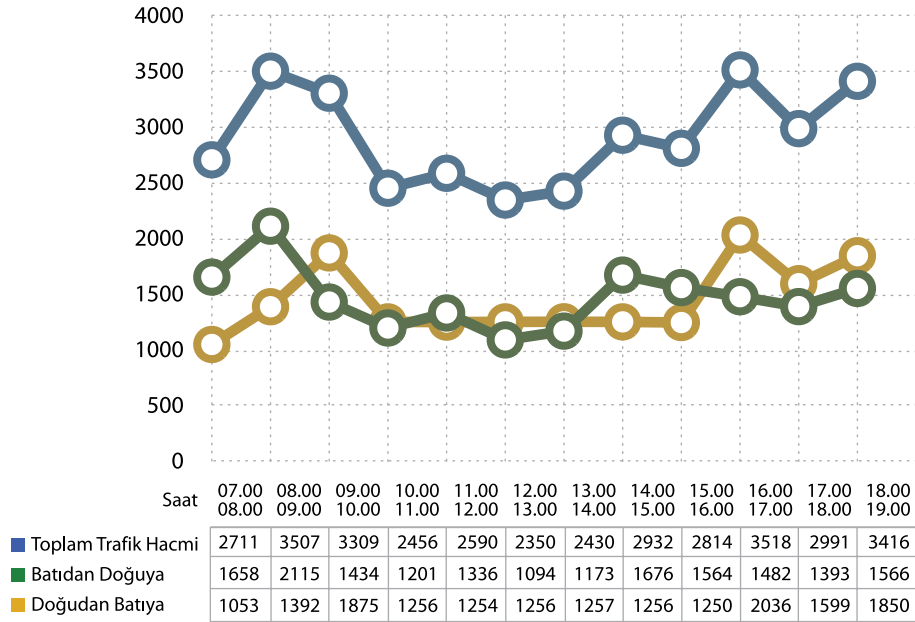
Batı-1 Perdesi Trafik Hacim Değerleri Grafiği
